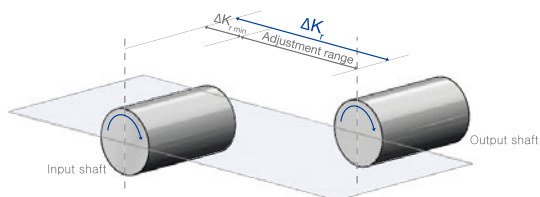
Figure 3. 반지름 방향 최대 허용 변위 (Maximum Radial Offset)
