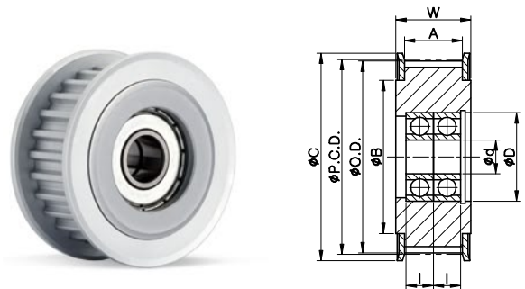
IDTC TYPE (Bearing 2 pcs.)
