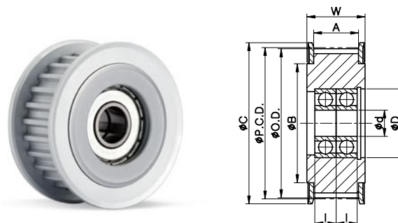
IDTC TYPE (Bearing 2 pcs.)
