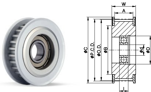
IDOC TYPE (Bearing 1 pc.)
