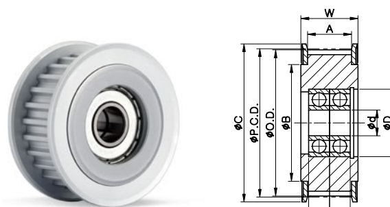
IDTC TYPE (Bearing 2 pcs.)
