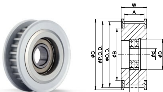
IDOC TYPE (Bearing 1 pc.)
