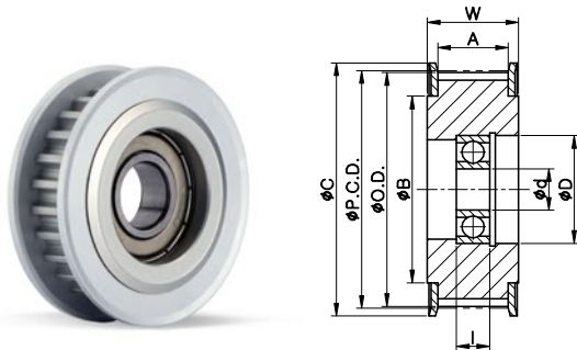
IDOC TYPE (Bearing 1 pc.)
